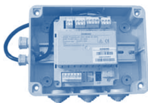
1 ks Externý modul AVS75 pre zmiešavaný vykurovací okruh vrátane 1 ks príložného čidla teploty QAD36/101
